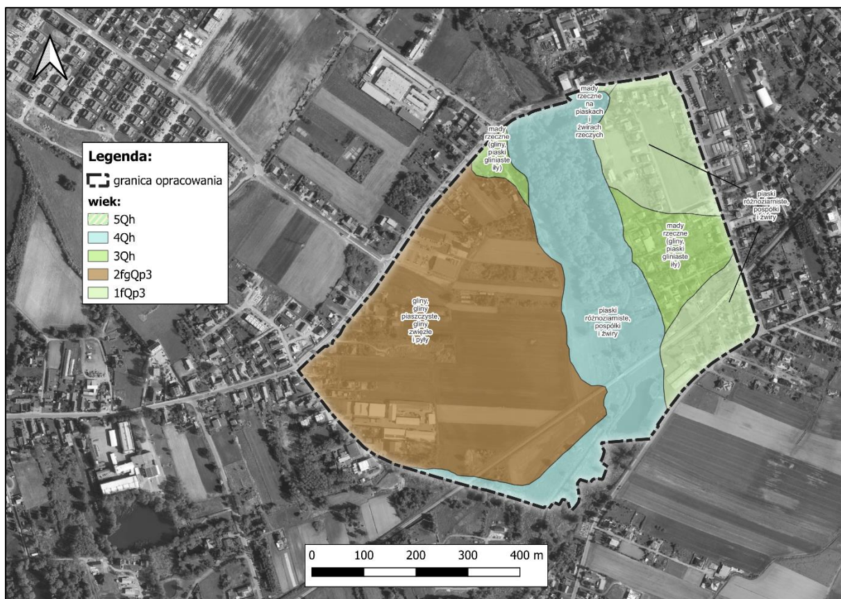
Rysunek 1 Warunki litologiczne
